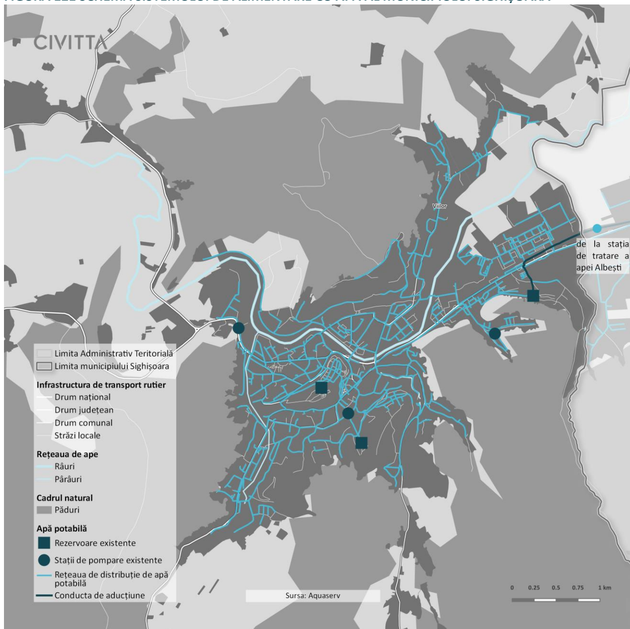
FIGURĂ 121 SCHEMA SISTEMULUI DE ALIMENTARE CU APĂ AL MUNICIPIULUI SIGHIȘOARA
